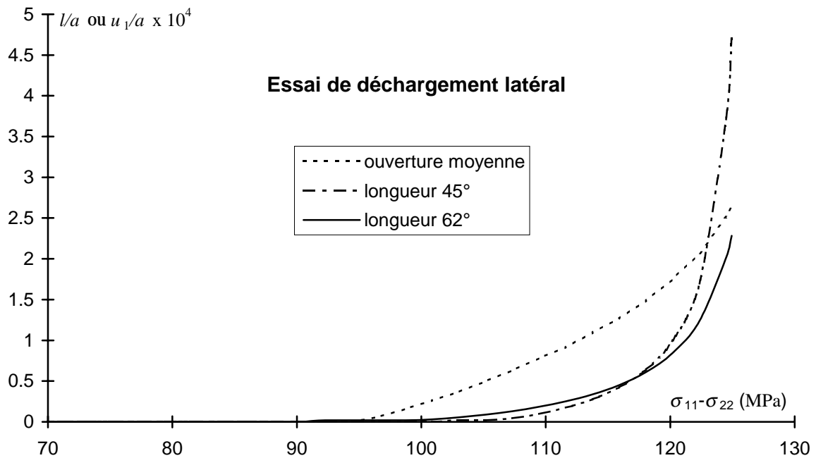
Figure IV.32 : Trajet de déchargement latéral : ouverture moyenne et longueur des branches.
