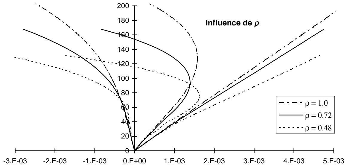
Figure AAnnexe 3.4 : Influence de la distribution de taille des mésolfissures initiales, \rho = \frac{a_0}{a_f} .
